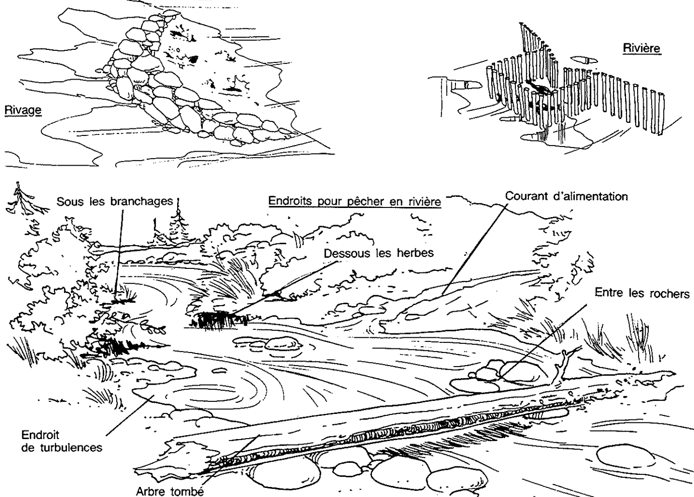
Fig. 20.18. Types de barrages à poissons
